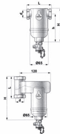
Вертикальное подсоединение
